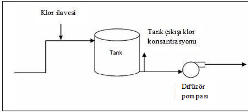
Şekil 1. Klorlama için örnek tank tasarımı
