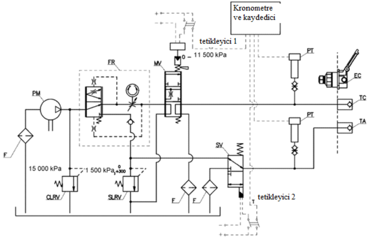
Şekil 2 - Traktör Simülatorü Hidrolik Şeması
