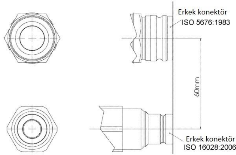
Şekil 1 - Hidrolik bağlantı devreleri
