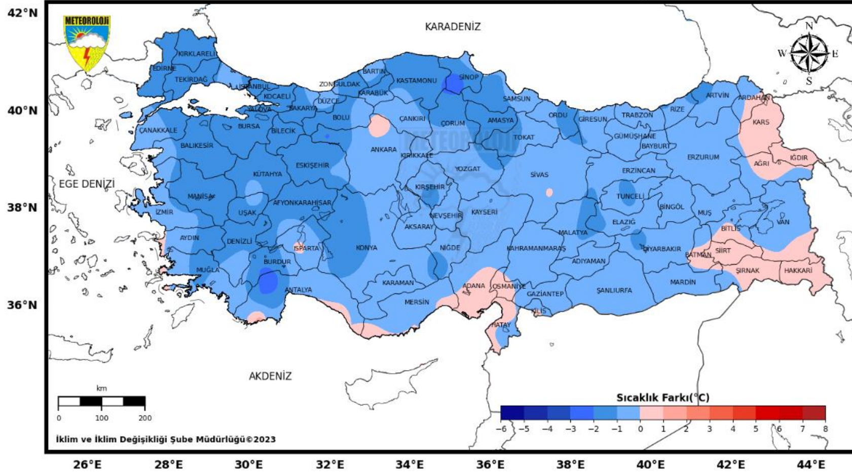
Şekil 1 Ortalama Sıcaklık Fark Haritası (Kaynak MGM: https://mgm.gov.tr/veridegerlendirme/sicaklik-analizi.aspx )
