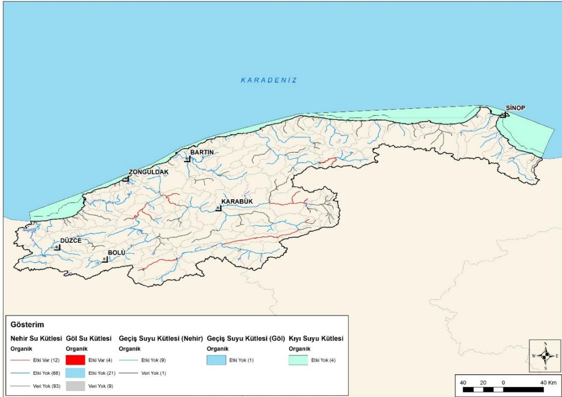
Şekil 3 Batı Karadeniz Havzasında organik kirlilik etkisi altındaki su kütlelerinin alansal temsili
